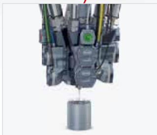
Präzisionsmischkopf MK 800 PRO mit Hochdruckwasserspülung
