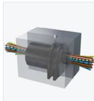
Die mit PU-Verguss ausgefüllte Form härtet bei Raumtemperatur oder zusätzlich durch das temperierte Formwerkzeug zur Kabeltülle aus.
