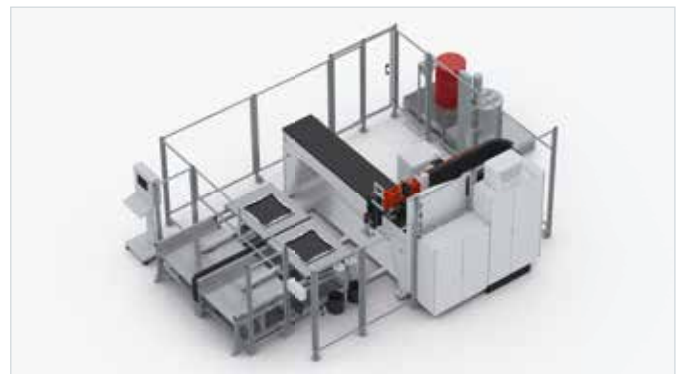
Alternative Prozessmöglichkeit: Misch- und Dosieranlage DM 502 mit 3-Achs-Linearroboter und Wechseltisch WT 1-LEVEL
