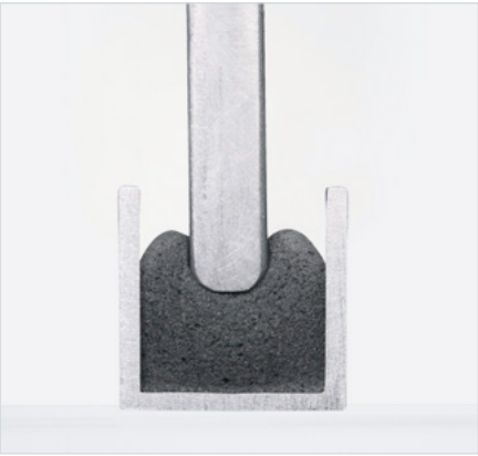
Querschnitt Polyurethanschaumraupe in Nut zu ca. 50 % verspresst
