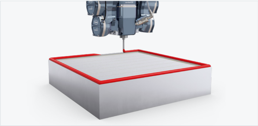
PU-Schaumauftrag mit CNC-gesteuertem Mischkopf auf ebenen Panelfilterrahmen
