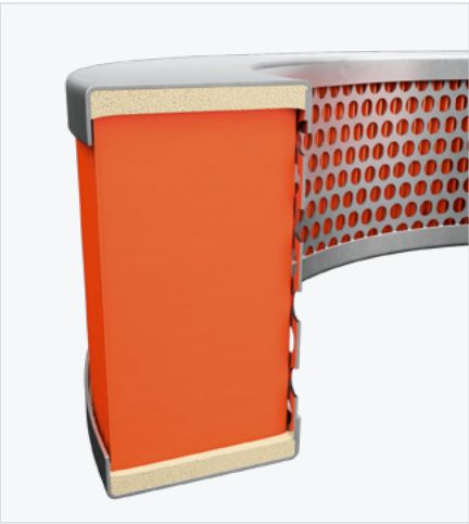
Querschnitt durch Radial-Luftfilter mit verklebten Endkappen (unten und oben)
